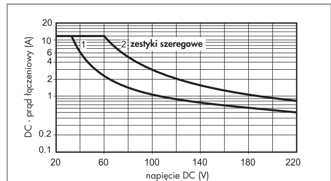
H 56 - Obciążenie graniczne dla prądu stałego (dla DC1) przy obciążeniu rezystancyjnym dla zestyków zwiernych, przerwa zestykowa \geq 1,5 mm
