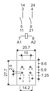
56.42-0300 rys. otworów montażowych
