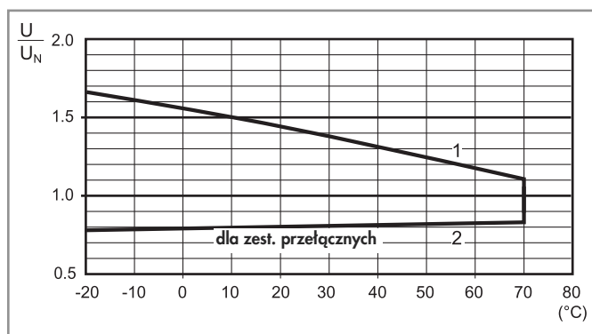
R 56 - AC Dopuszczalny zakres napięcia pracy cewki w zależności od temperatury otoczenia, 4 zestyki przełączne (4P)
