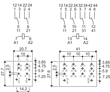
56.42 rys. otworów montażowych
